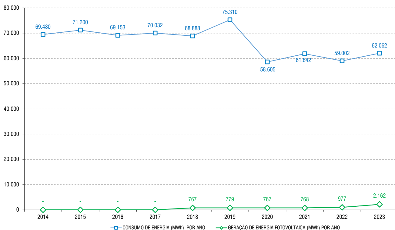
Gráfico 17.2 - CONSUMO DE ENERGIA E GERAÇÃO DE ENERGIA FOTOVOLTAICA - 2014 A 2023
