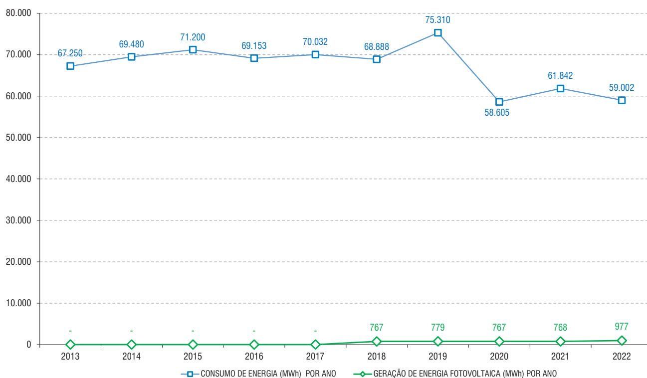
Gráfico 17.2 - CONSUMO DE ENERGIA E GERAÇÃO DE ENERGIA FOTOVOLTAICA
