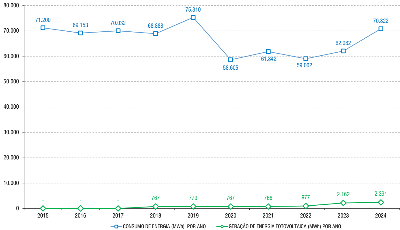
Gráfico 17.2 - CONSUMO DE ENERGIA E GERAÇÃO DE ENERGIA FOTOVOLTAICA - 2015 A 2024
